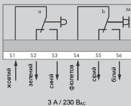
Схема підключення додаткових контактів NESM...-15S
