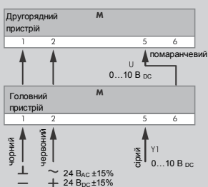
Схема підключень NESM24.2-15(S) Паралельне підключення
