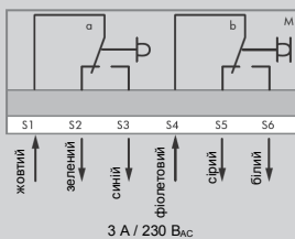
Схема підключення додаткових контактів NESM...-10S
