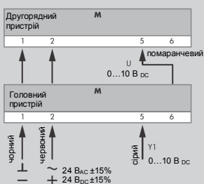
Схема підключень NESM24.2-10(S) Паралельне підключення
