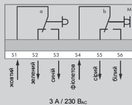
Схема підключення додаткових контактів NESM...-03S
