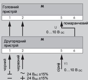
Схема підключень NESM24.2-03(S) Паралельне підключення
