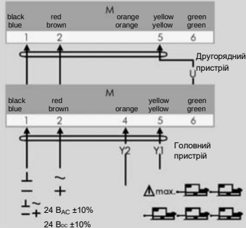
Схема підключень NABM 1.2-10 (S1)
