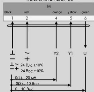
Схема підключень NABM 1.2-10 (S1) Живлення 24 В AC / DC
