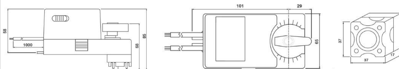
РОЗМІРИ СЕРВОПРИВОДА [мм]
